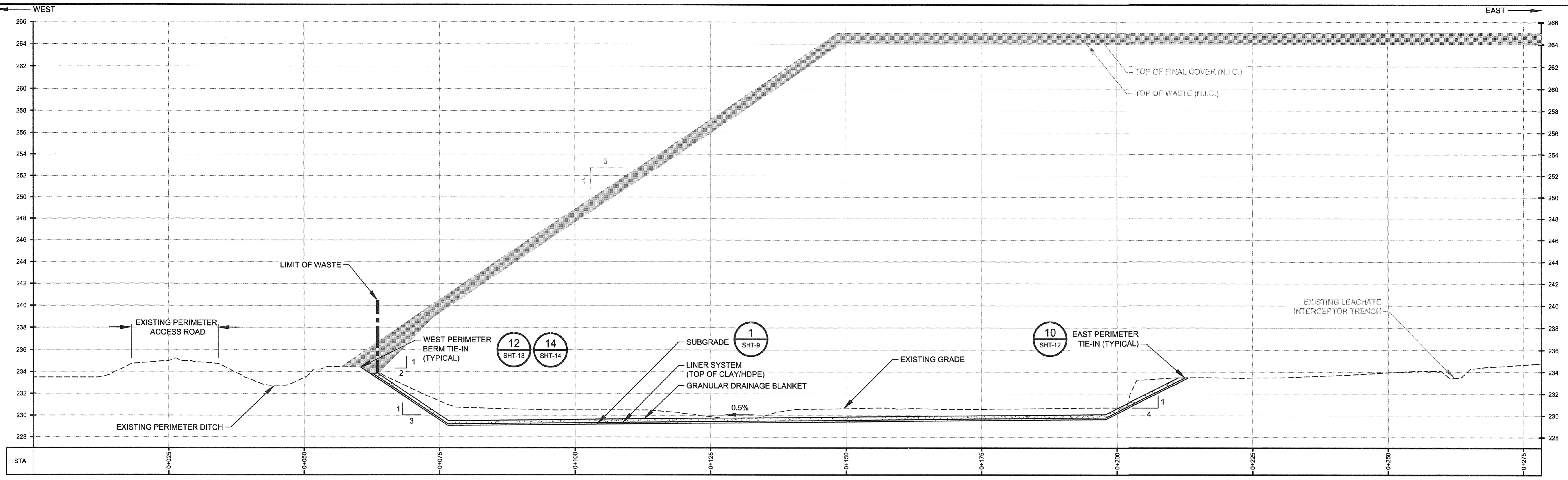
SECTION A-A VERT: 1:200 HORIZ: 1:400 SHT-5
