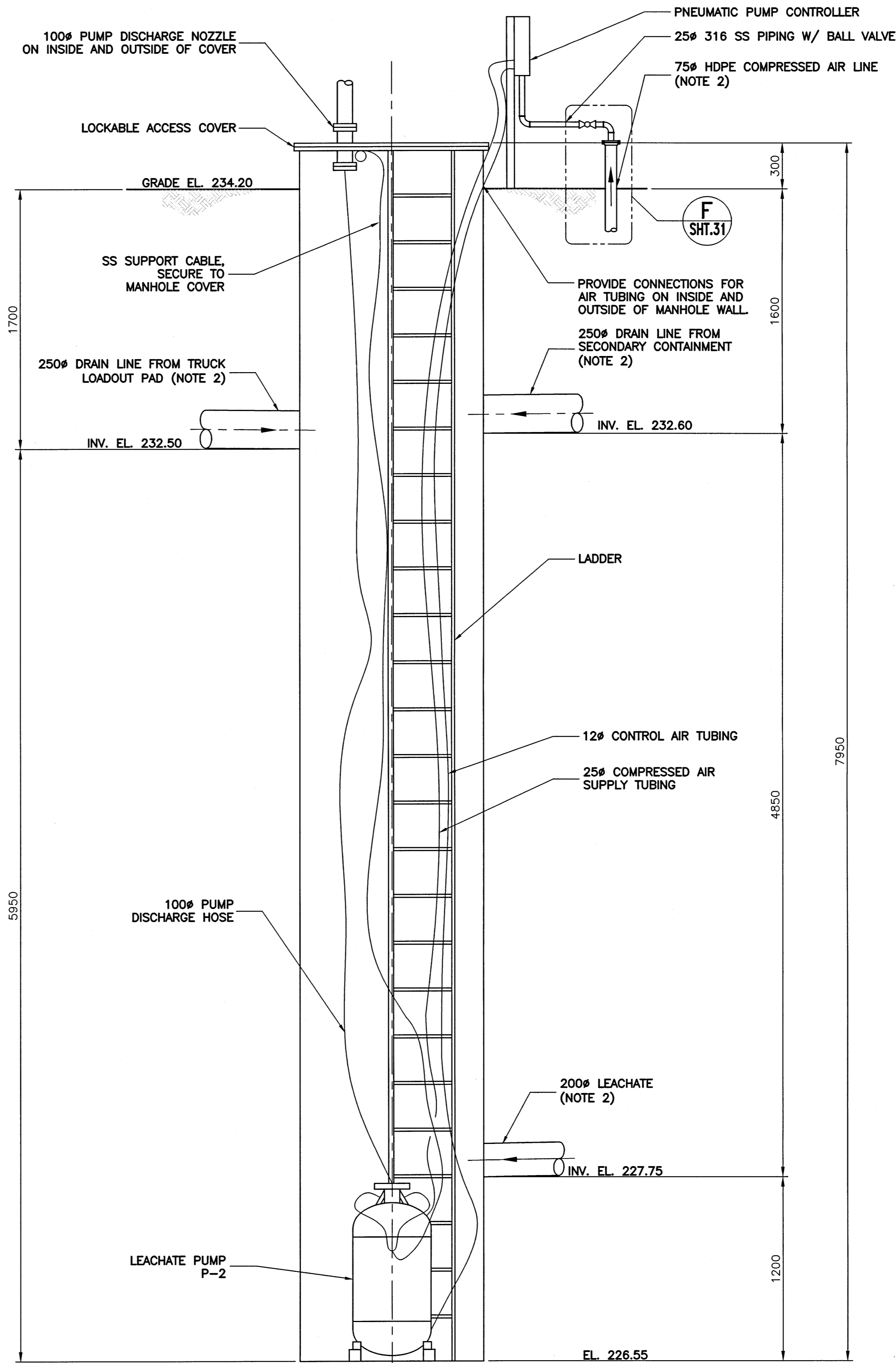
2 MANHOLE MH03 - ELEVATION
