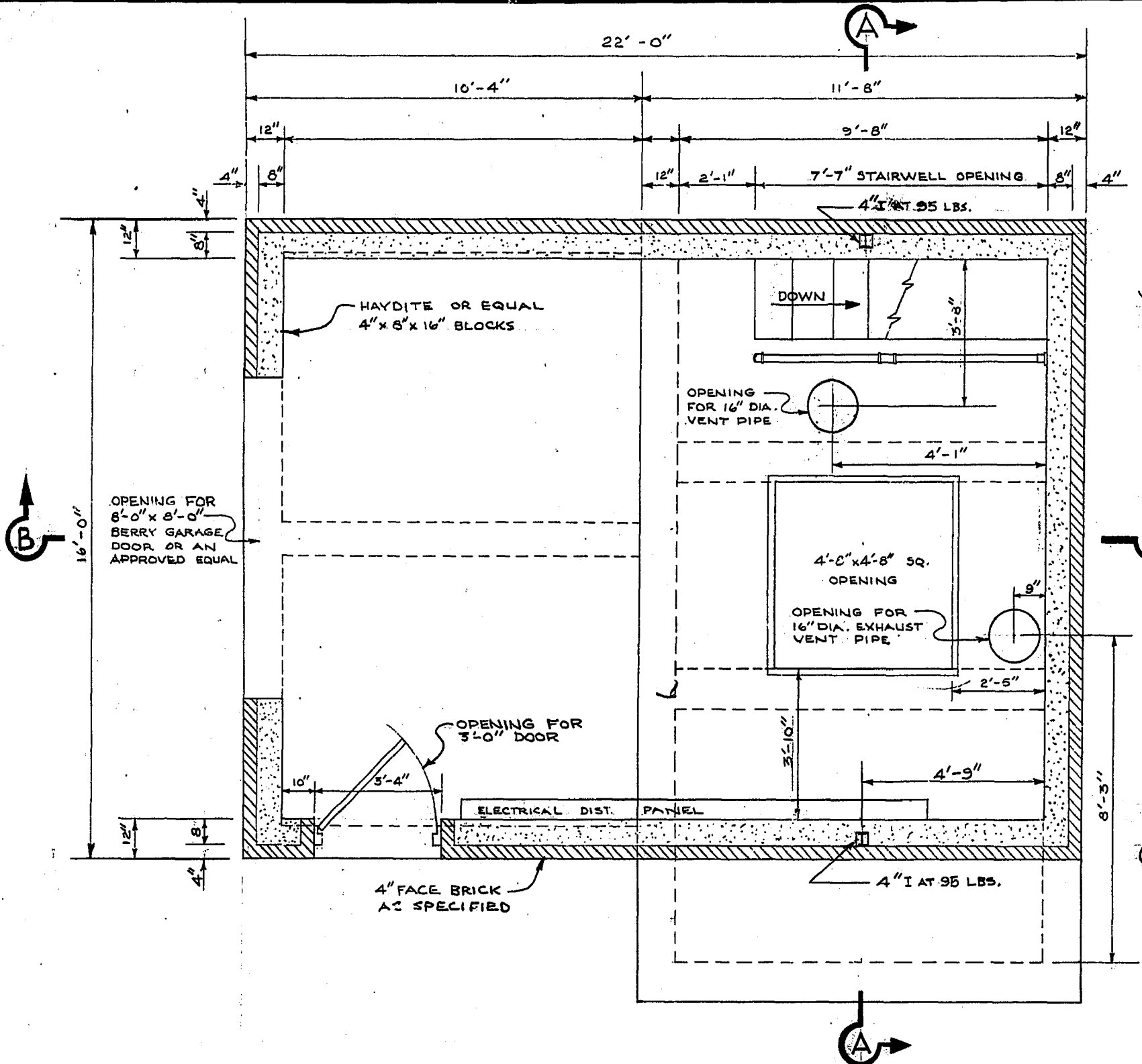
FLOOR PLAN SCALE: 3/8" = 1'-0"
