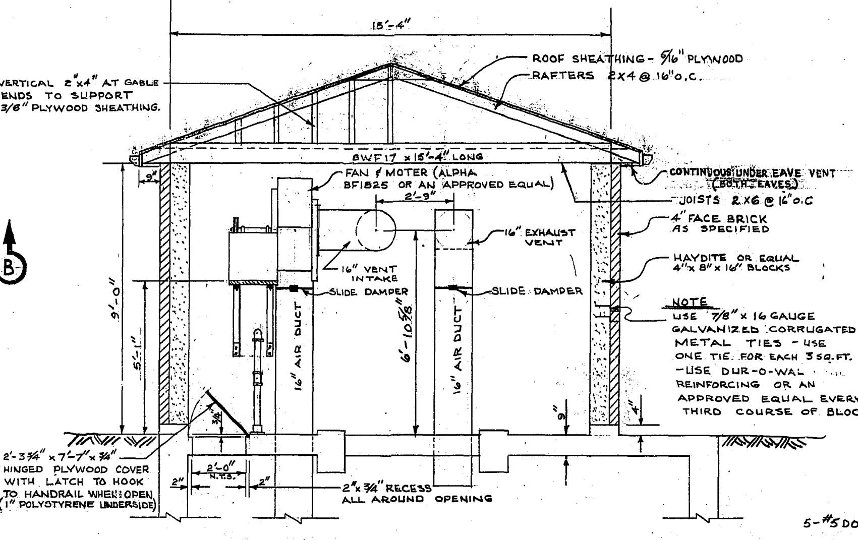
SEC. "A-A" SCALE: 3/8" = 1'-0"
