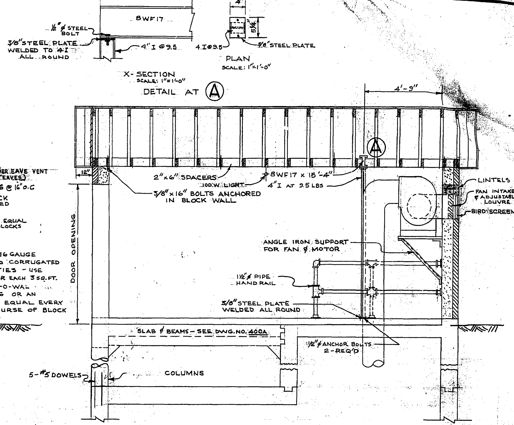
SEC. "B-B" SCALE: 3/8" = 1'-0"
