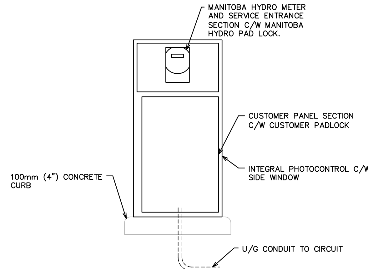
2 METERED ELECTRICAL PANEL DETAIL E1.1 SCALE: N.T.S.
