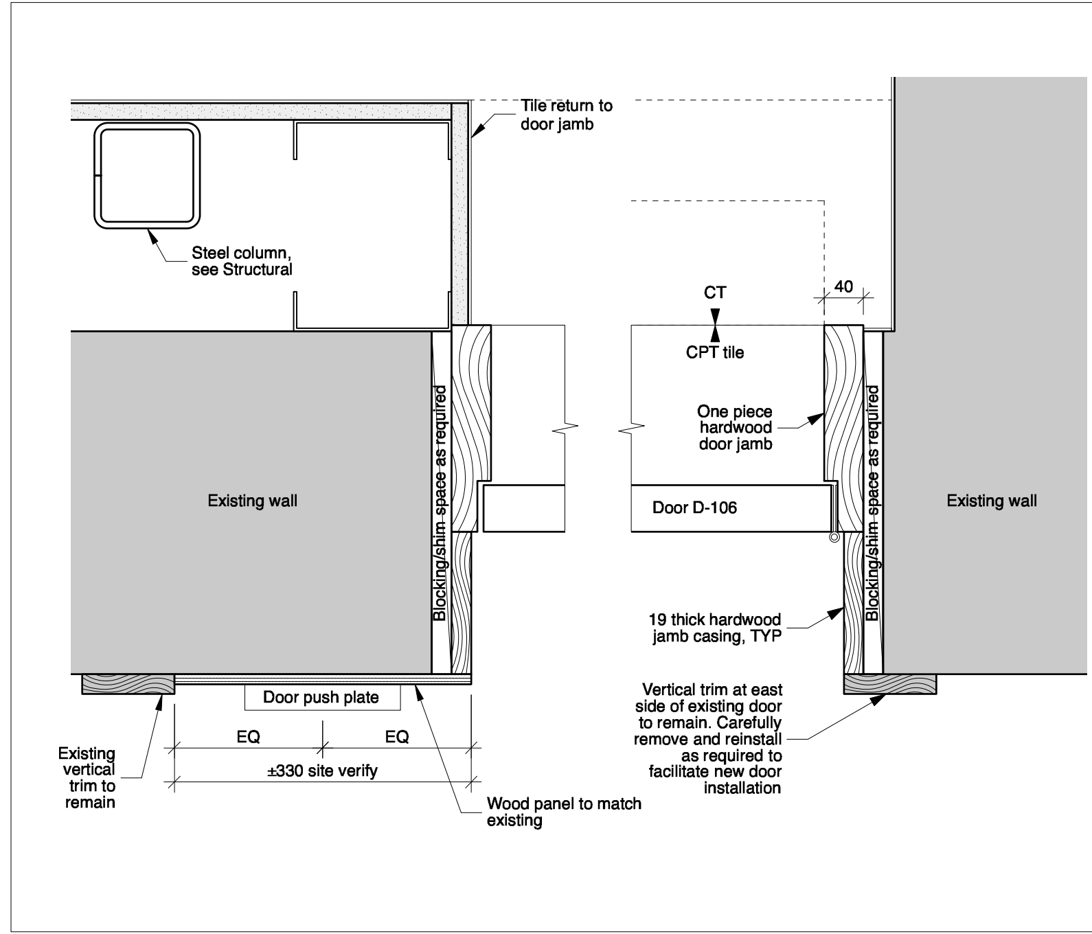
10 Plan Detail - Door D-106 Jamb A-700 1:5
