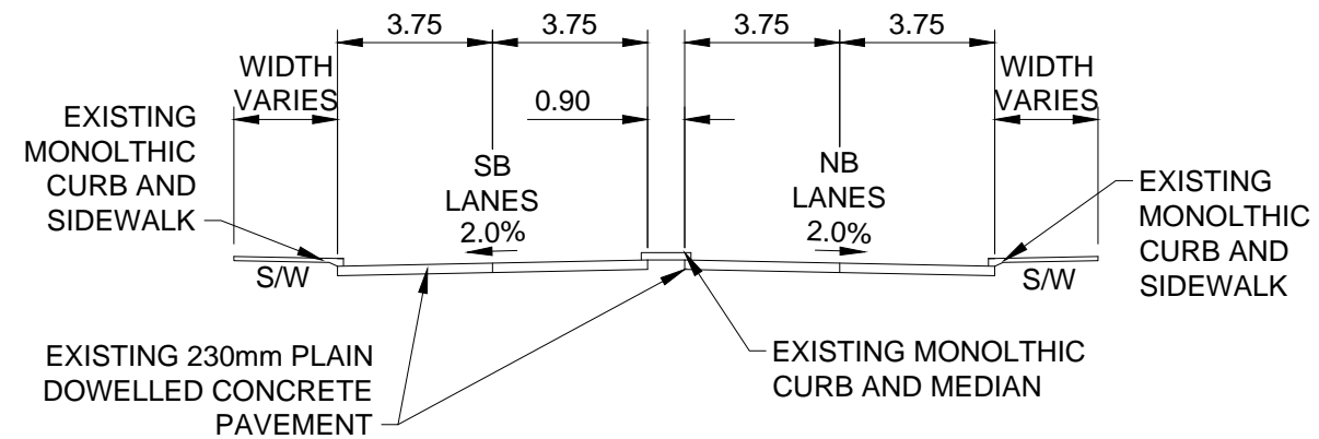
A TYPICAL SECTION N.T.S.
