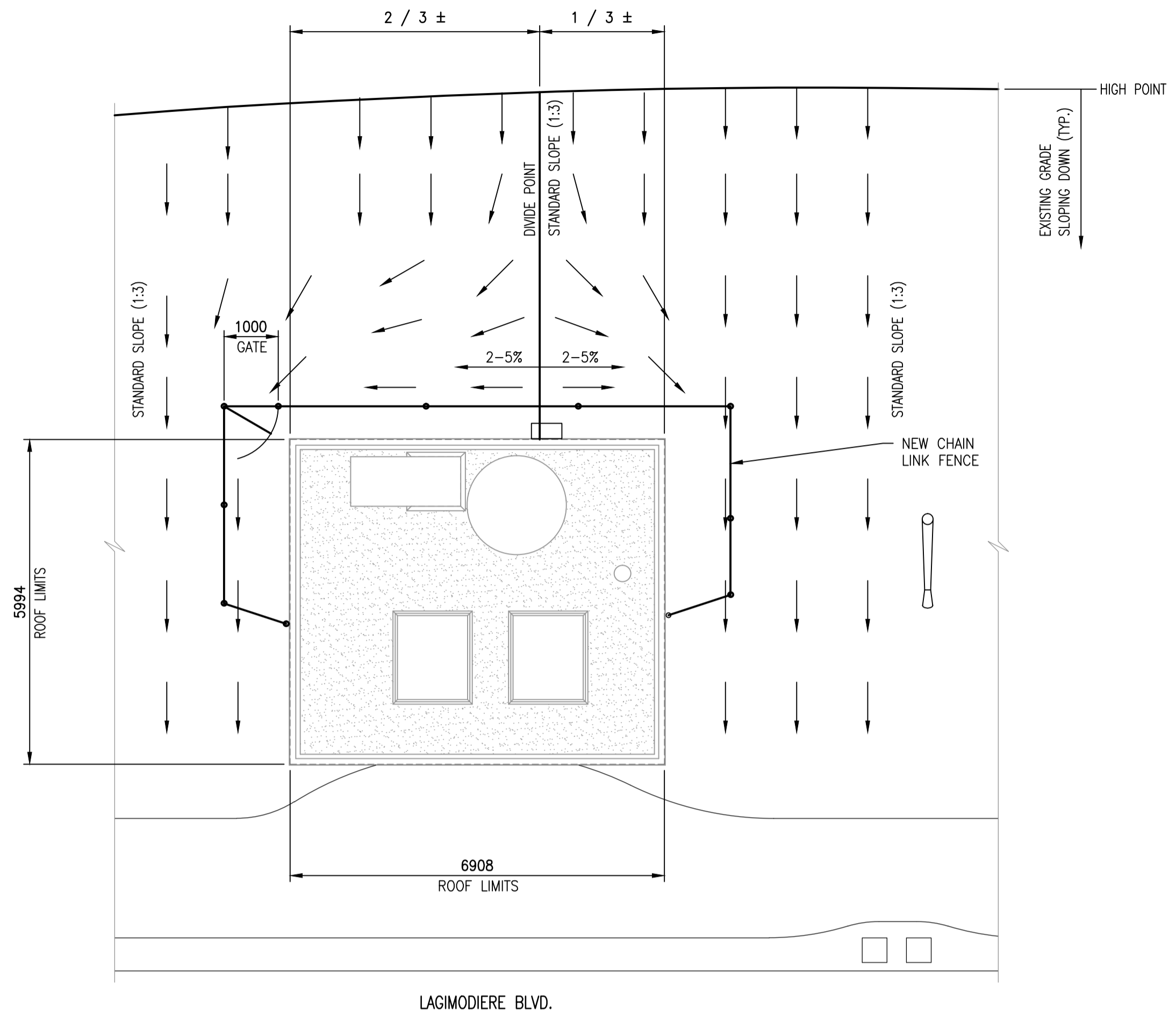
SITE PLAN - GRADING 1 : 75
