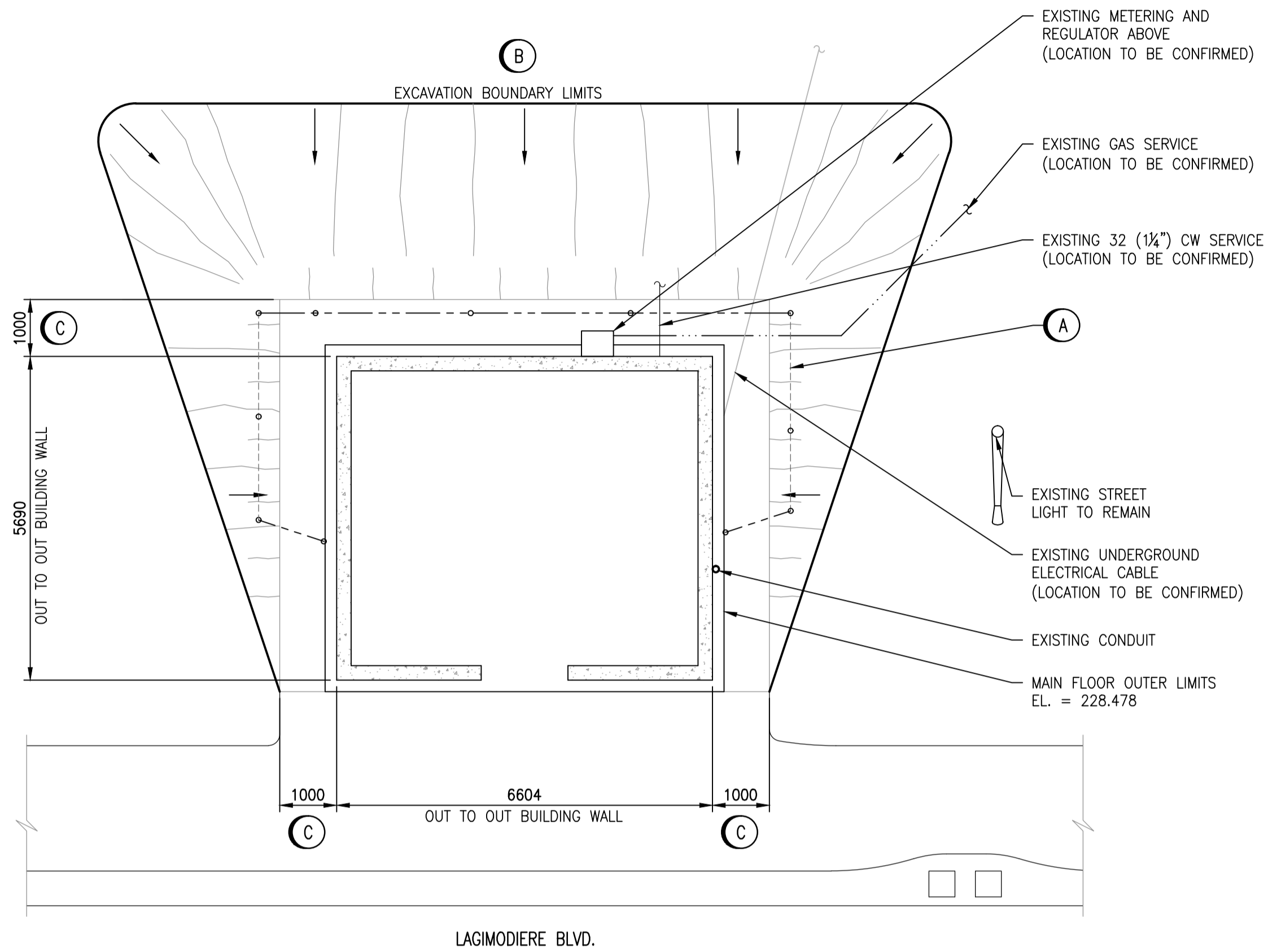
SITE PLAN - EXCAVATION 1 : 75
