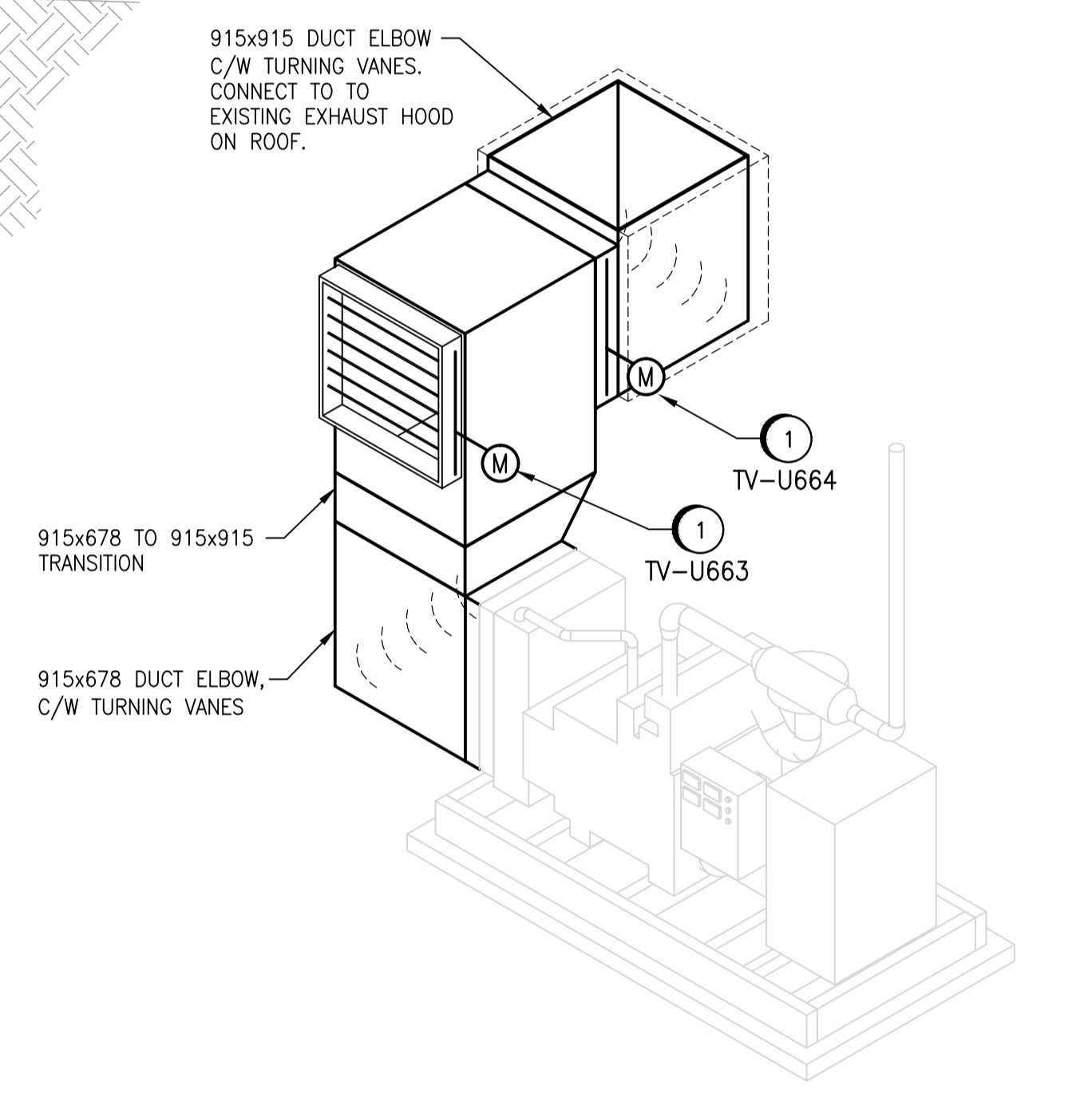
GENERATOR COOLING EXHAUST ISOMETRIC SCALE: N.T.S.
