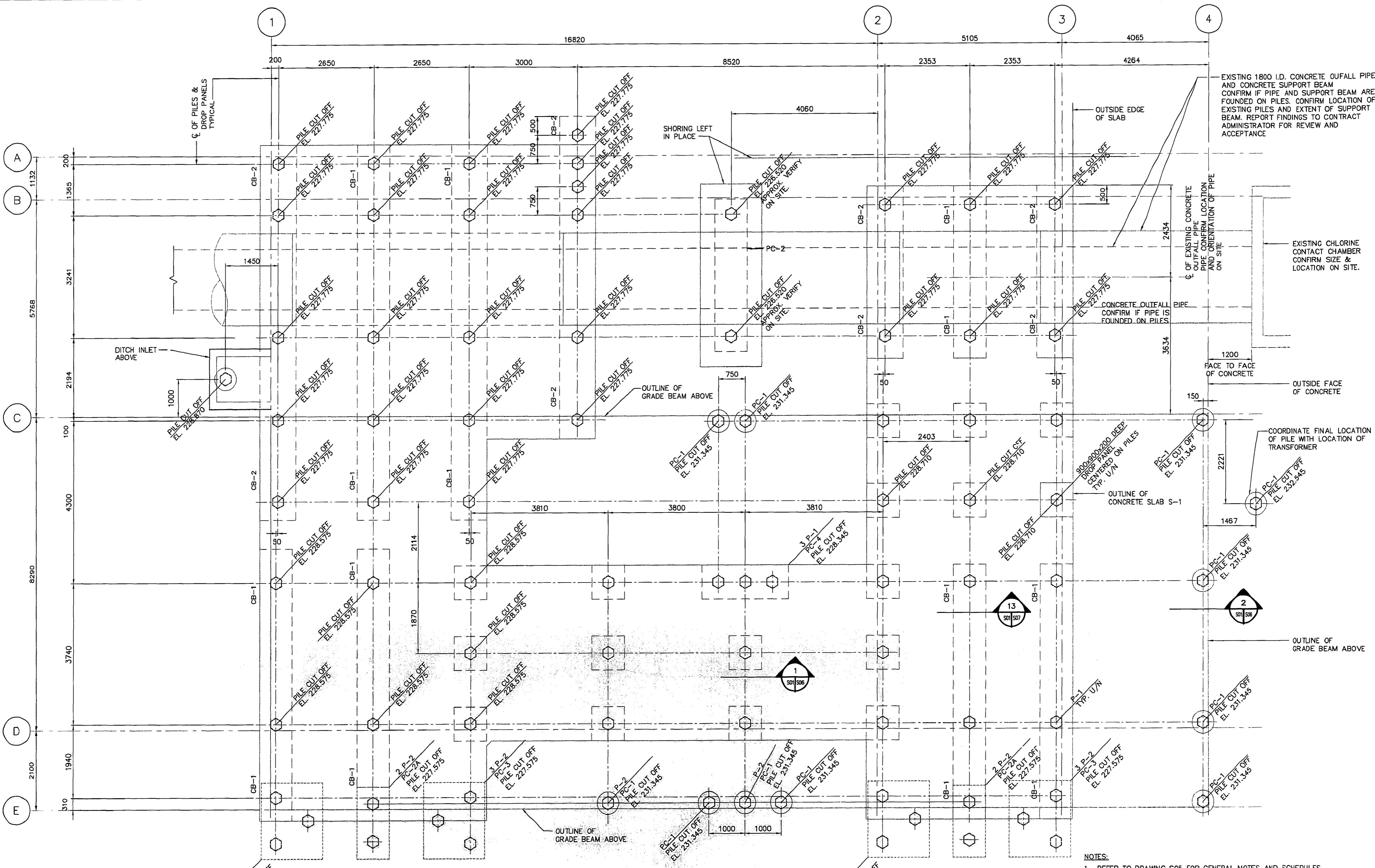
PILING PLAN SCALE: 1:50
