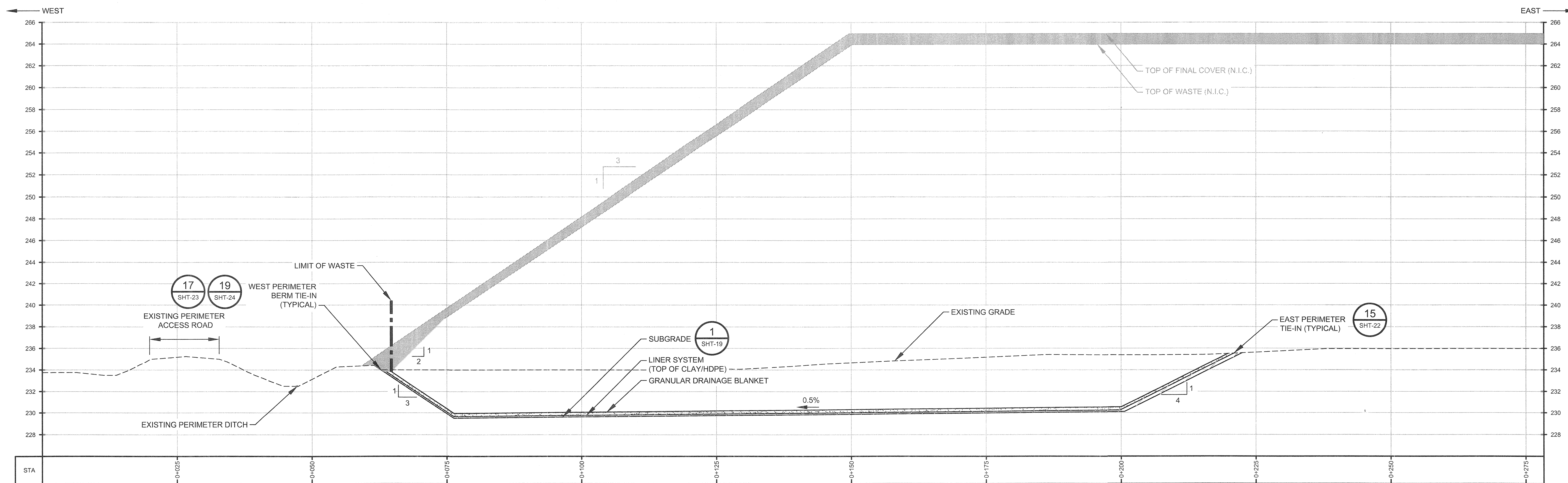
SECTION A-A' VERT: 1:200 HORIZ: 1:400 SHT-6
