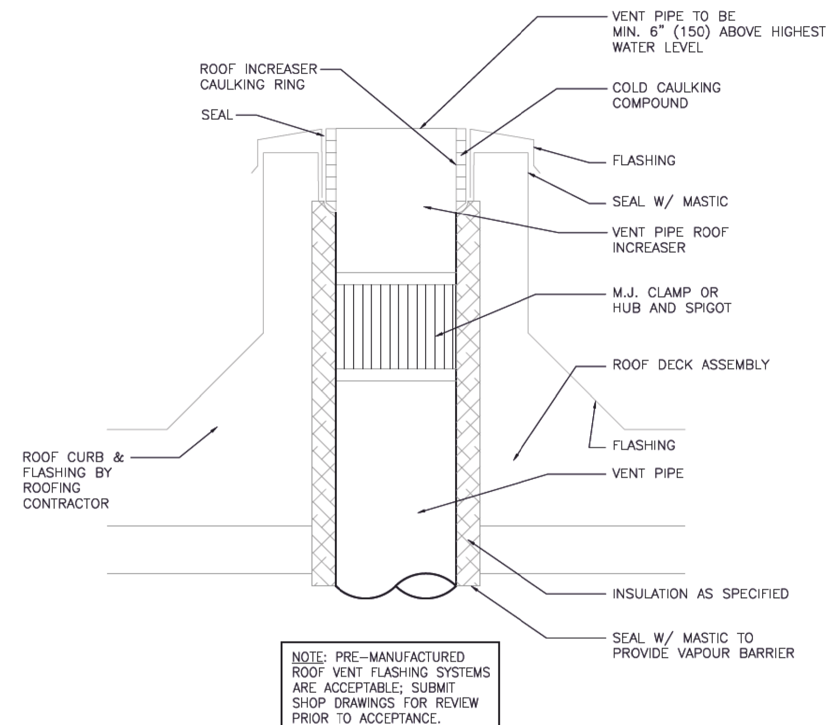
PLUMBING VENT DETAIL SCALE: N.T.S.
