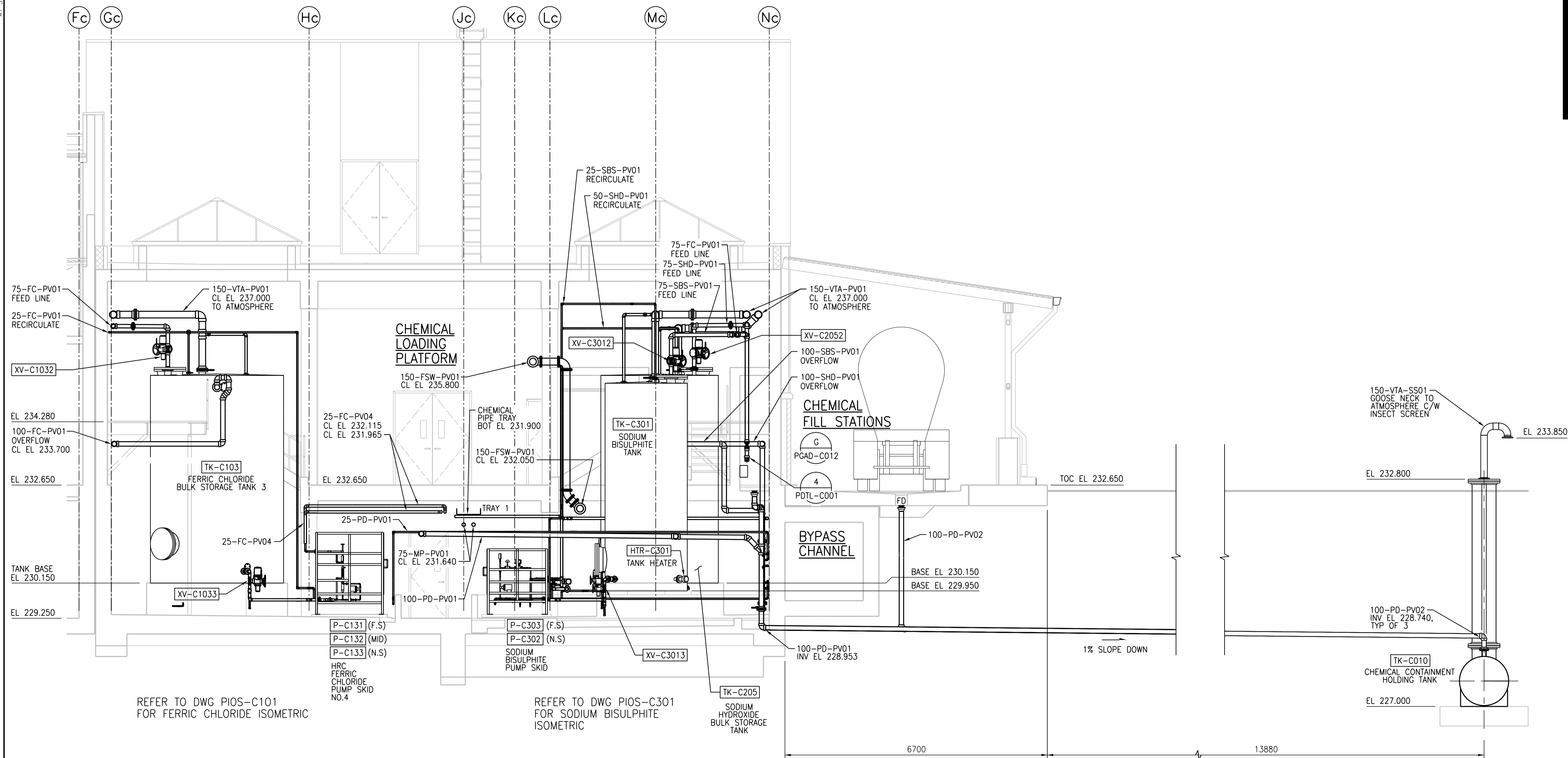
E SECTION 1:50 PGAD-C002 PGAD-C003
