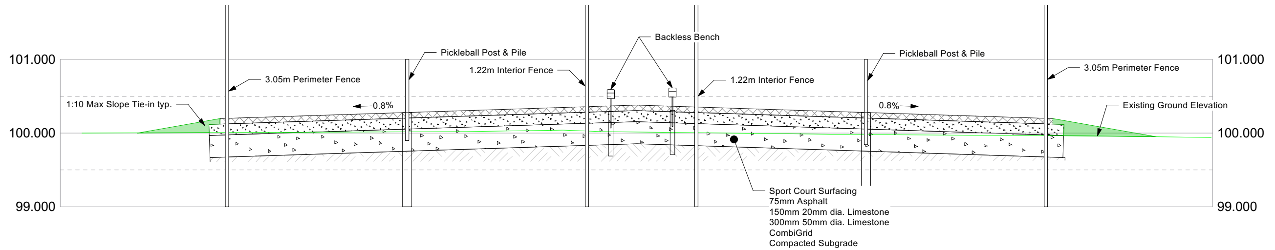
1-A COURT PROFILE N-S
