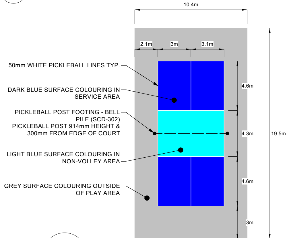
2-A COURT DETAILS TYP.
