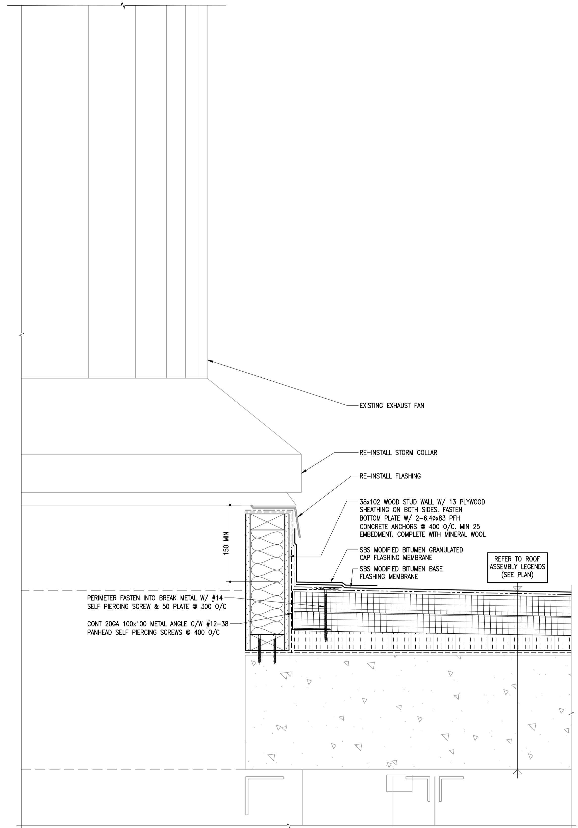
2 EXHAUST FAN DETAIL 1-0601B-00076-008 1:5
