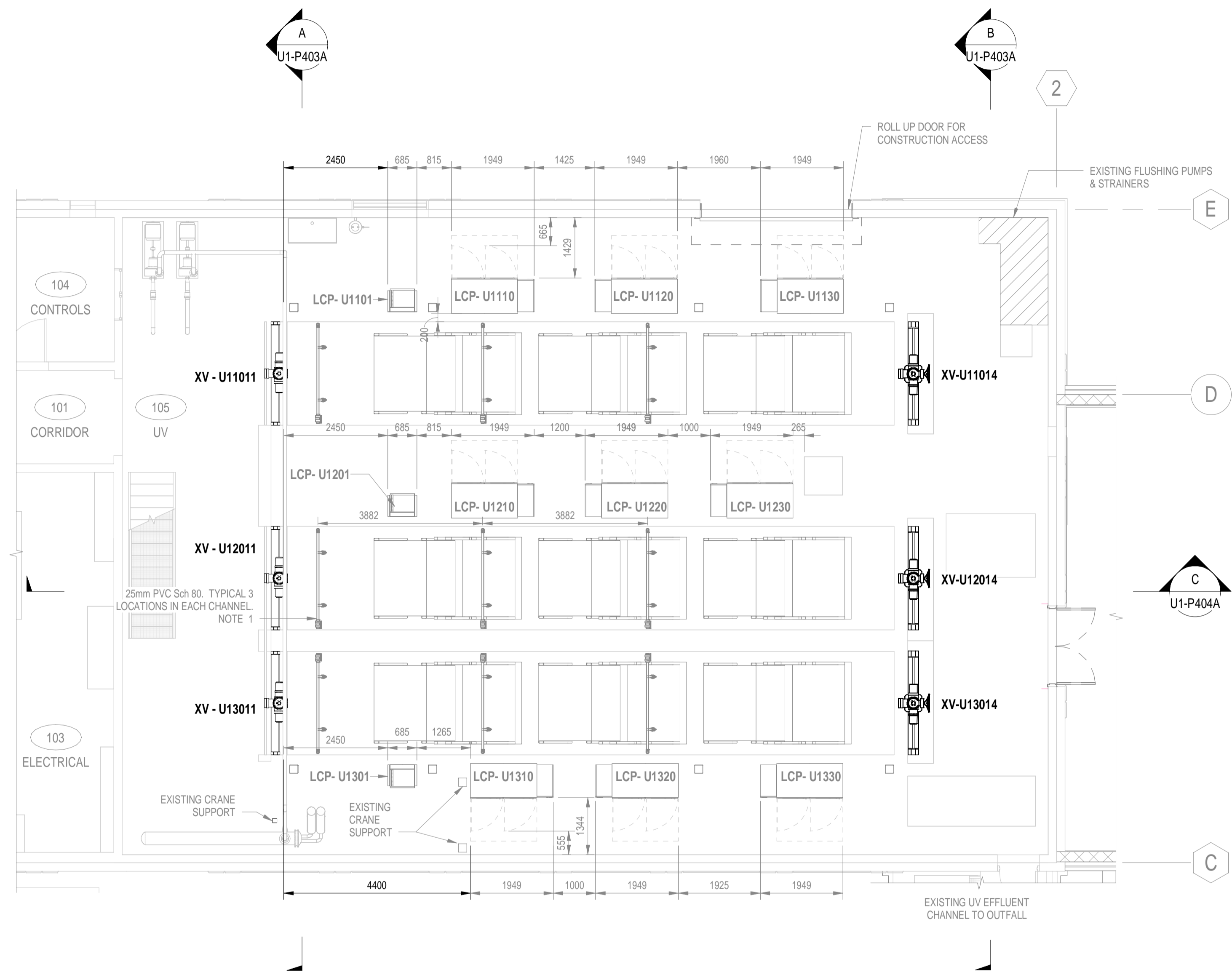
1 | PLAN AT EL 237.000m SCALE: 1 : 75
