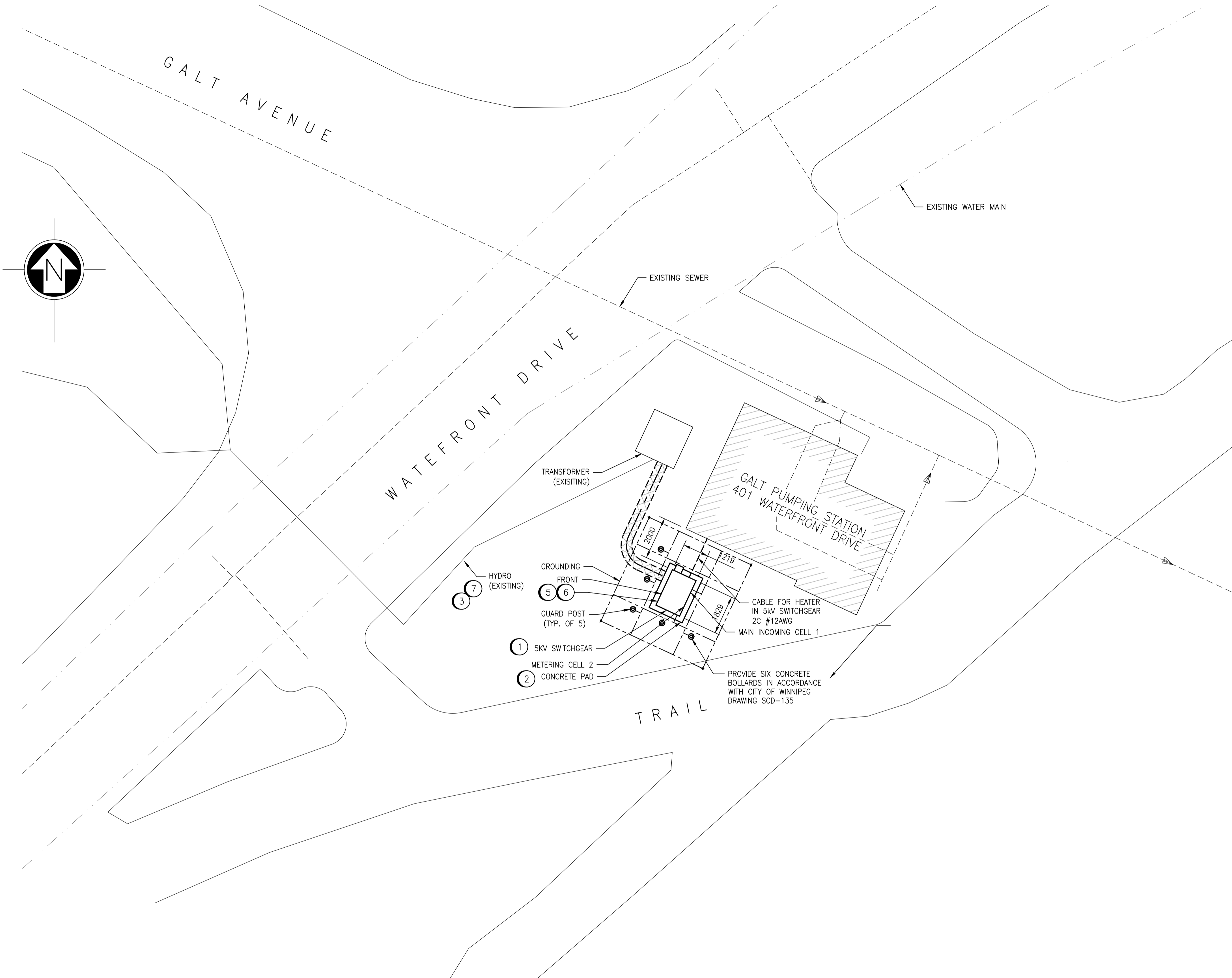
ELECTRICAL SITE PLAN SCALE: 1 : 100
