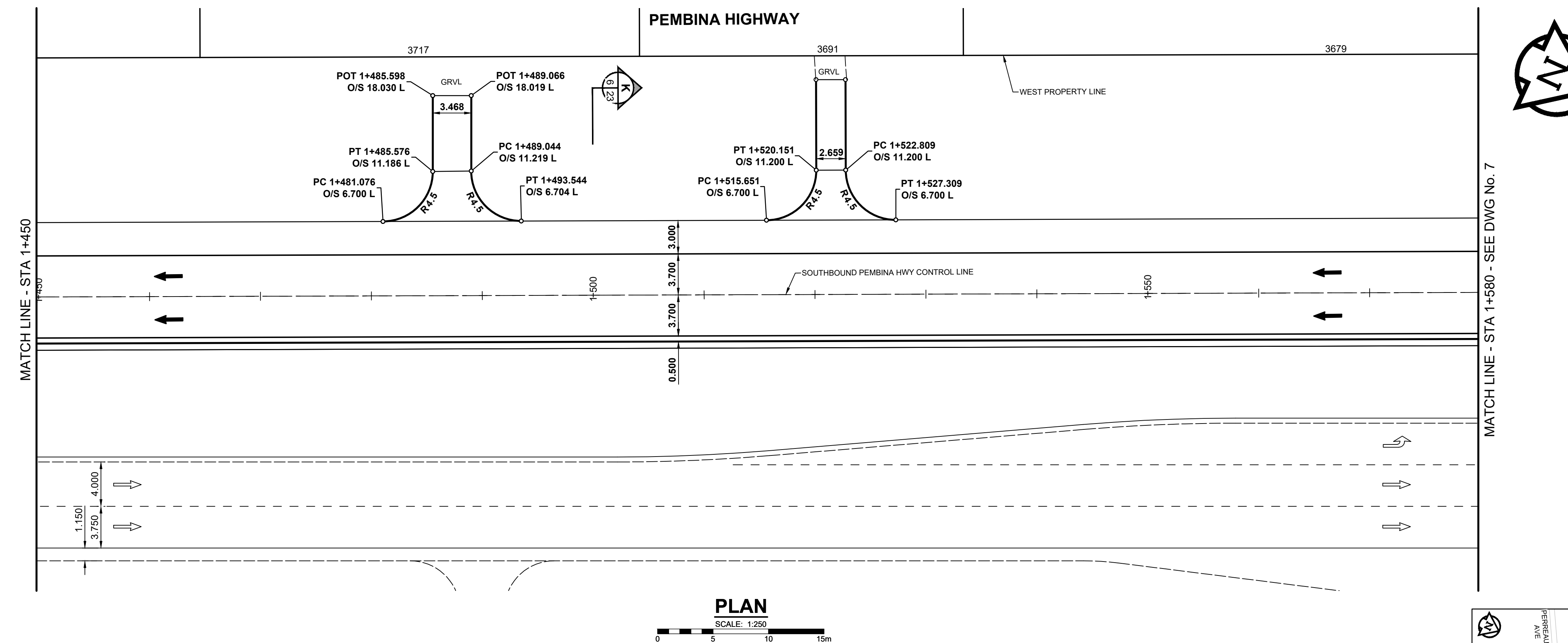
PLAN SCALE: 1:250 0 5 10 15m
