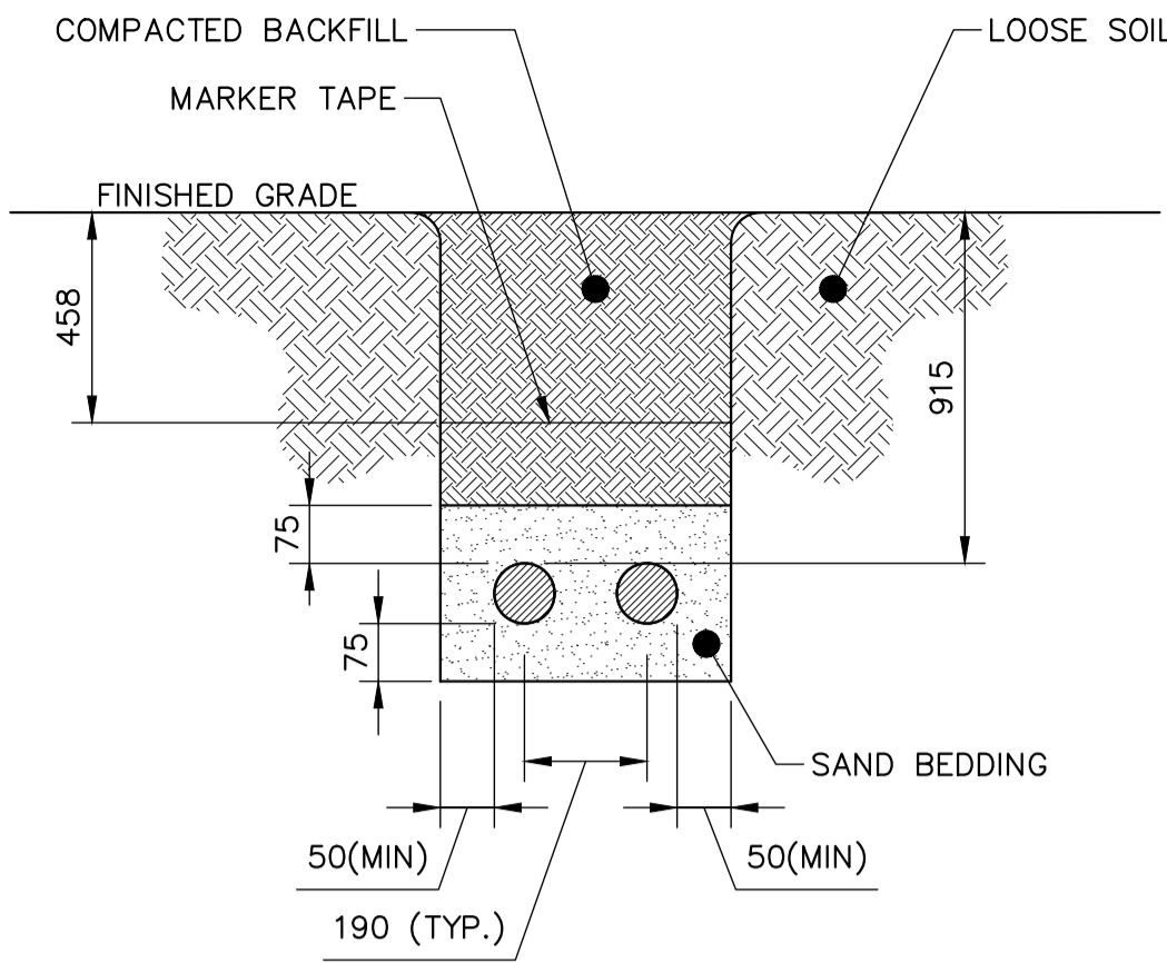
3 CABLE TRENCH DETAIL – 2 CABLES SCALE: N.T.S.
