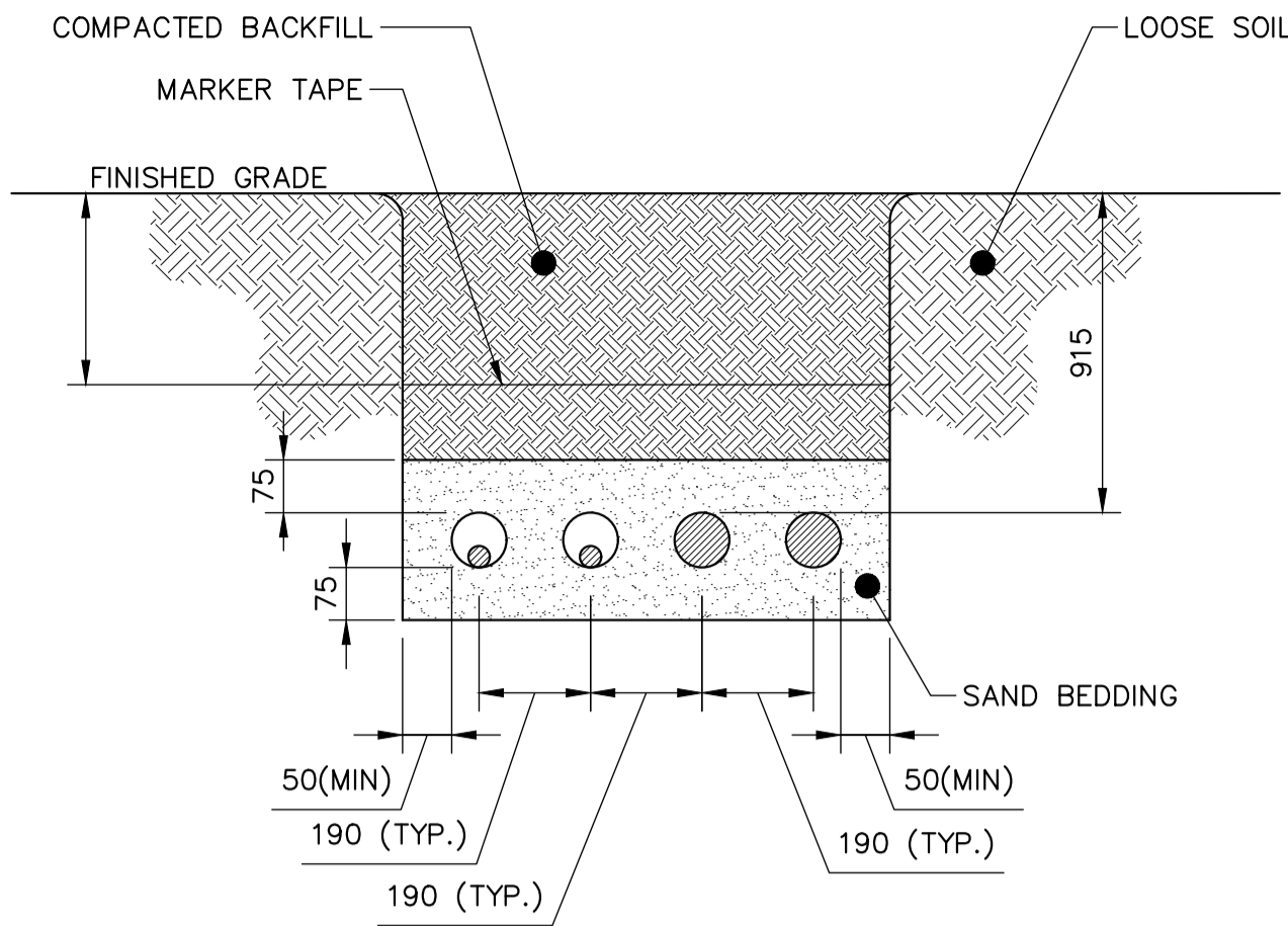
2 CABLE TRENCH DETAIL – 4 CABLES SCALE: N.T.S.
