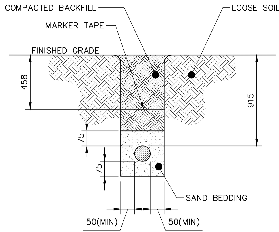
1 CABLE TRENCH DETAIL – 1 CABLE SCALE: N.T.S.
