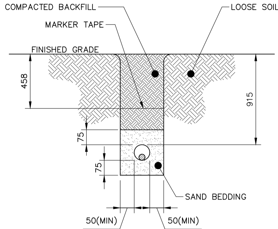
4 CABLE TRENCH DETAIL – 1 CABLE SCALE: N.T.S.
