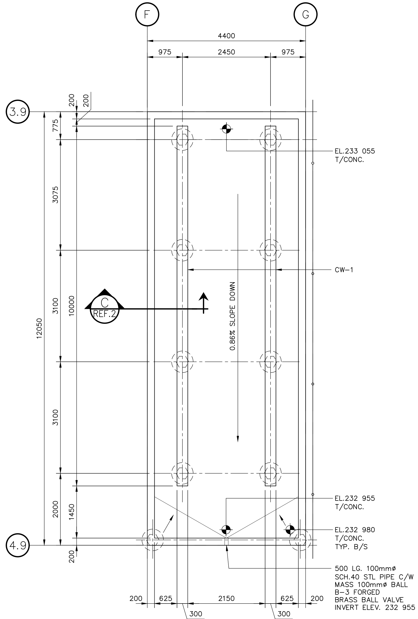
2 DETAIL REF.1 SCALE: 1:50
