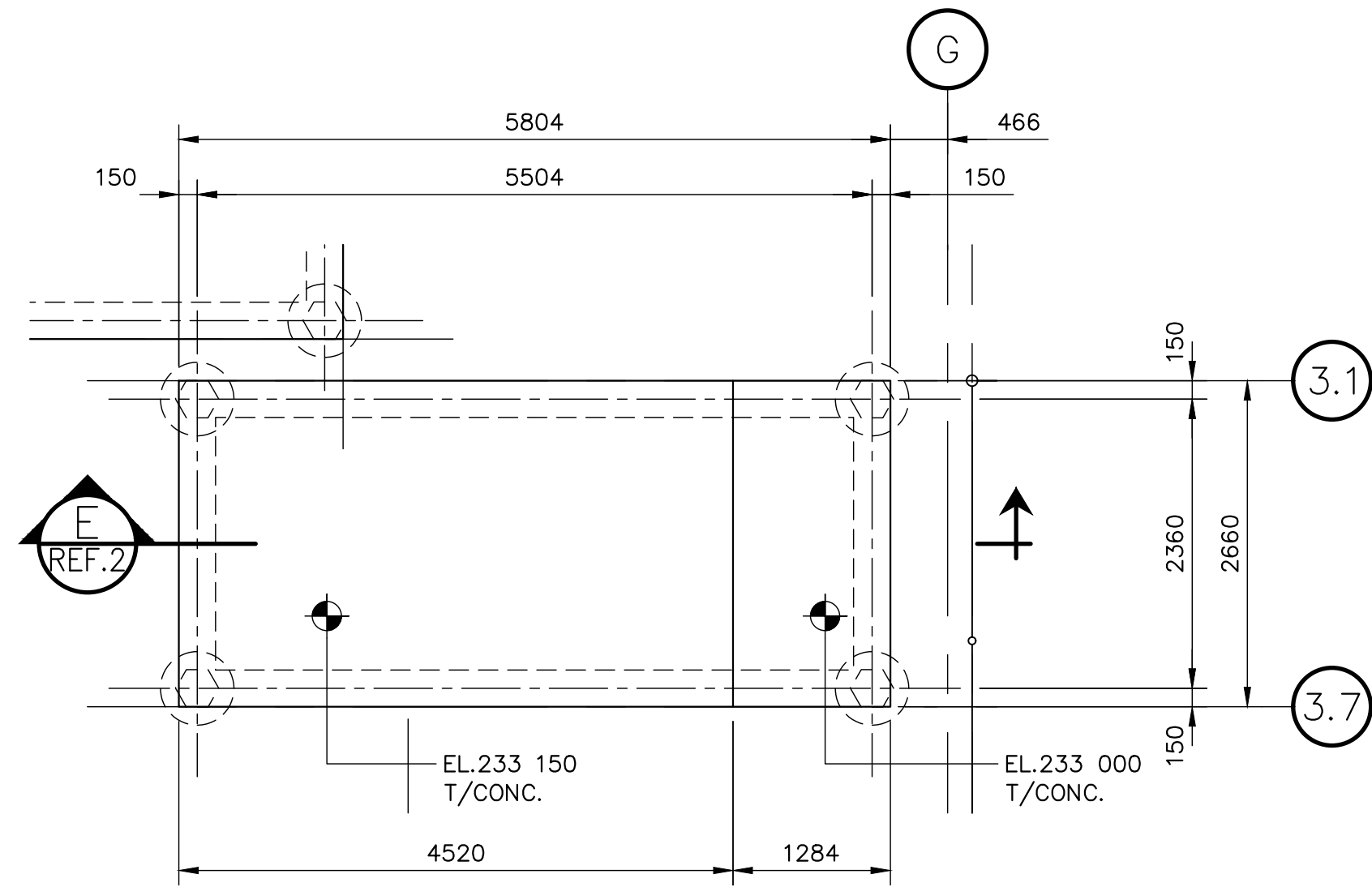
1 DETAIL REF.1 SCALE: 1:50
