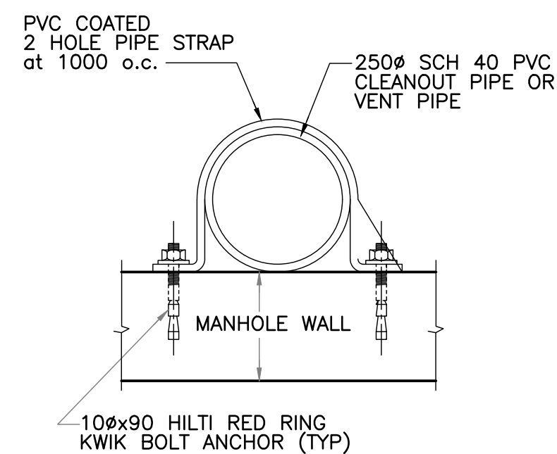
DETAIL D – PIPE STRAP SCALE: N.T.S.
