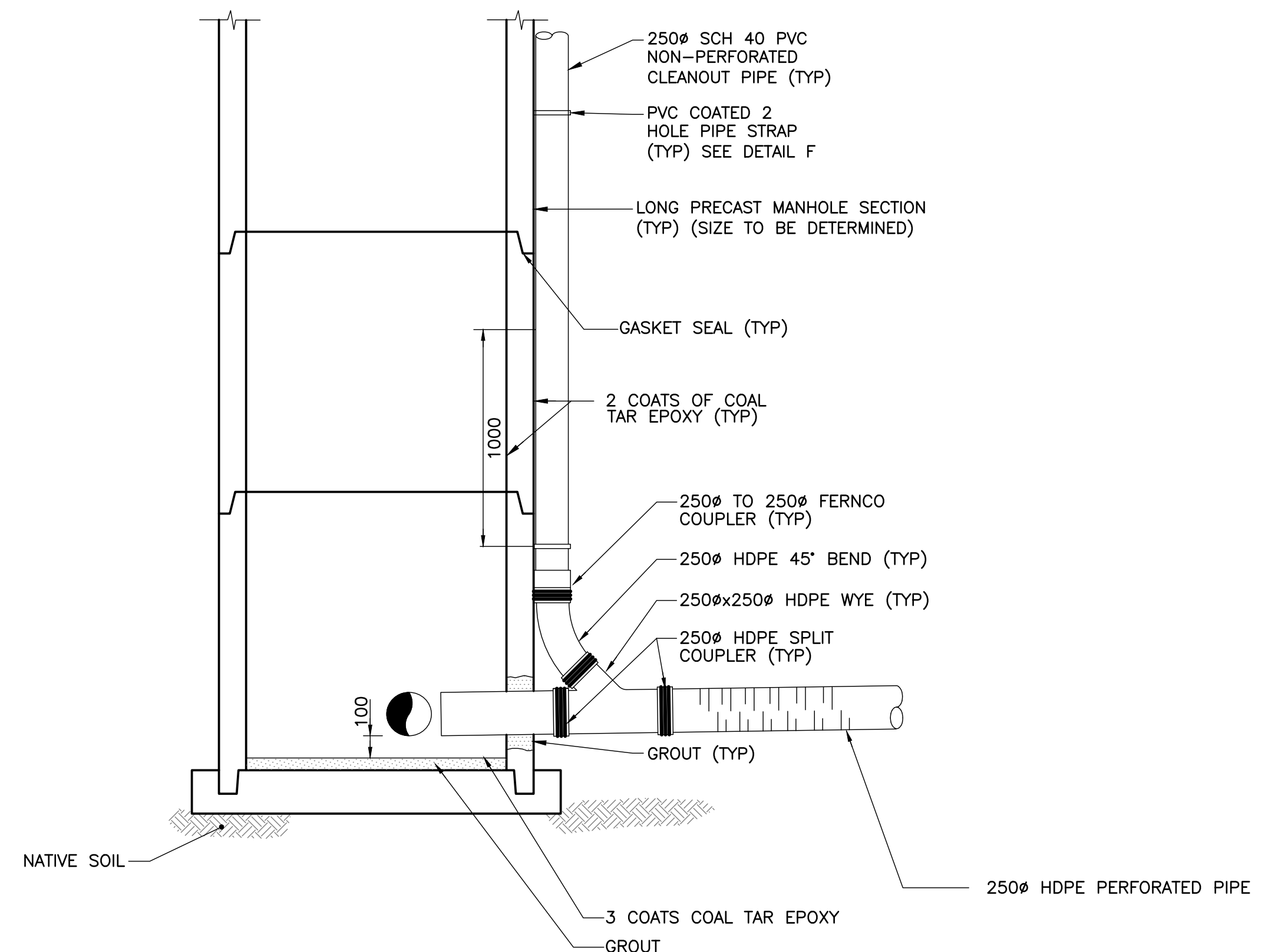
SECTION 2 – SIDE VIEW SCALE: N.T.S.
