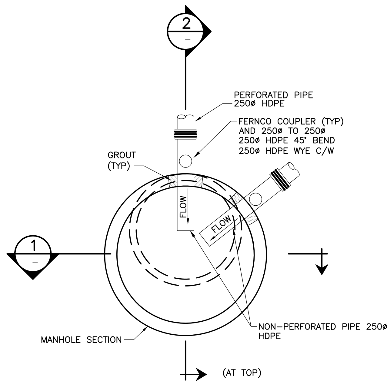
DETAIL C – PLAN VIEW SCALE: N.T.S.
