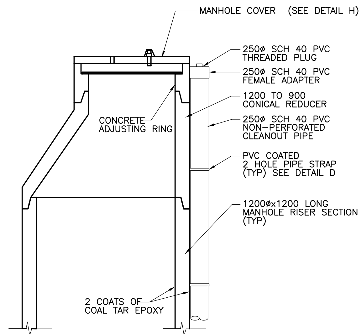
SECTION 1 – FRONT VIEW SCALE: N.T.S.
