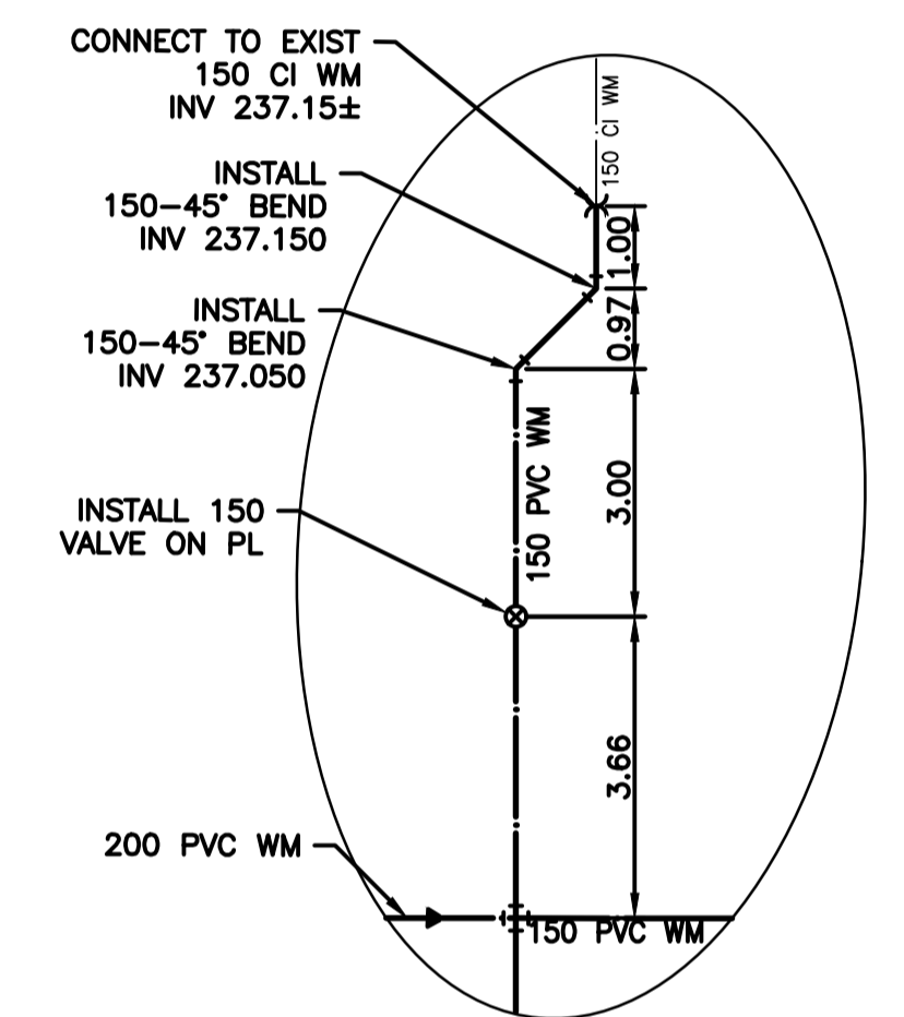
DETAIL "A" SCALE: NTS
