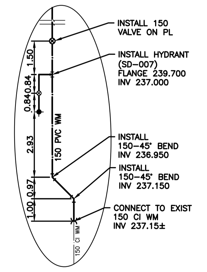
DETAIL "B" SCALE: NTS
