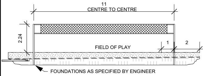
CROSS SECTION SCALE: 1:180
